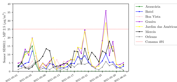
Figura 3.1: Médias diárias de MP_{2,5} dos pontos de amostragem para maio de 2021.
