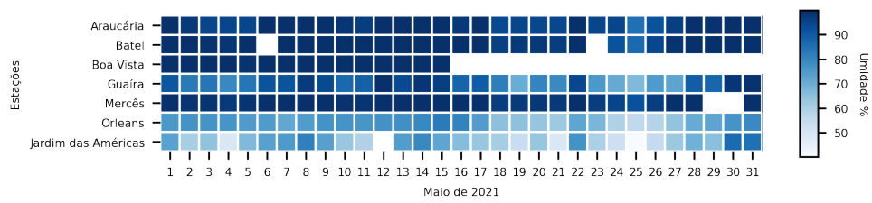
Figura 3.8: Umidade média diária nos pontos amostrais
