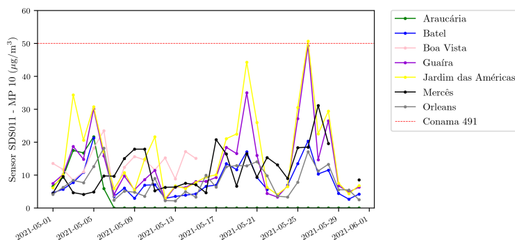
Figura 3.2: Médias diárias de MP_{10} dos pontos de amostragem para maio de 2021.
