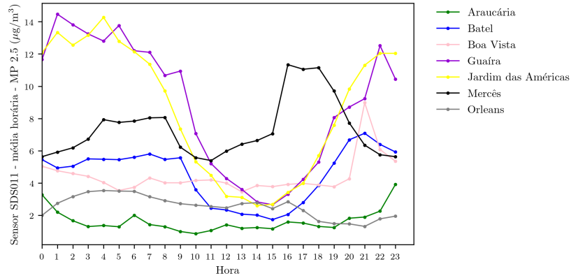
Figura 3.3: Perfis diários de MP 2,5 dos pontos de amostragem para maio de 2021
