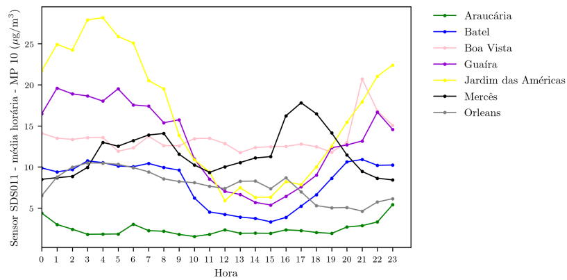
Figura 3.4: Perfis diários de MP 10 dos pontos de amostragem para maio de 2021
